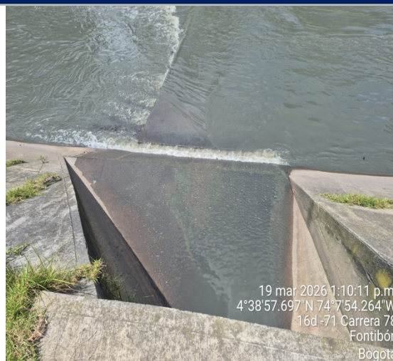
Fotografías 1 y 2. El punto corresponde a la inspección realizada el 19/03/2026 a la estructura de descarga Red Troncal Pluvial AK 72 con código RFU-T4-0051.
